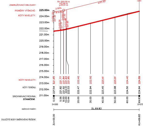
ŘEZ OSOU IV
