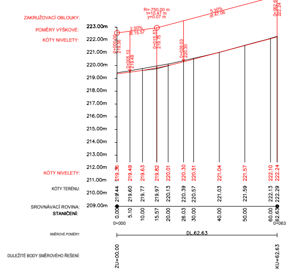
ŘEZ OSOU II
